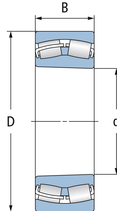
Kegelige Bohrung Tapered bore
