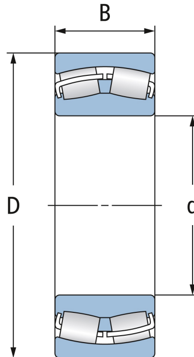
Zylindrische Bohrung Cylindrical bore
